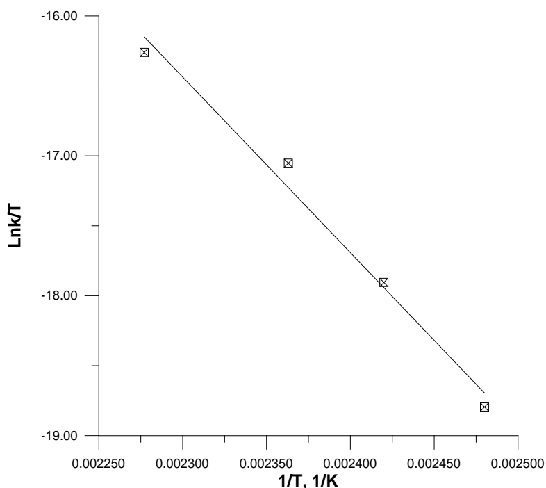
Figura 3. Representación de Eyring, correspondiente a la reacción de descomposición térmica del DPAG en solución de metanol
