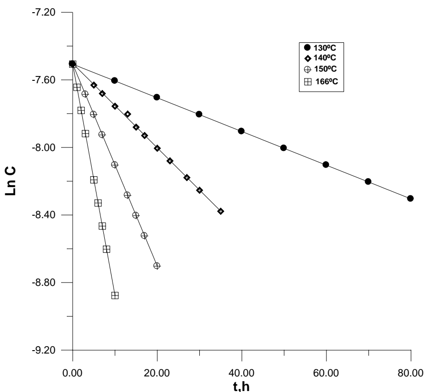
Figura 2. Representación gráfica de la cinética de primer orden de los datos obtenidos de la termólisis del DPAG en metanol
